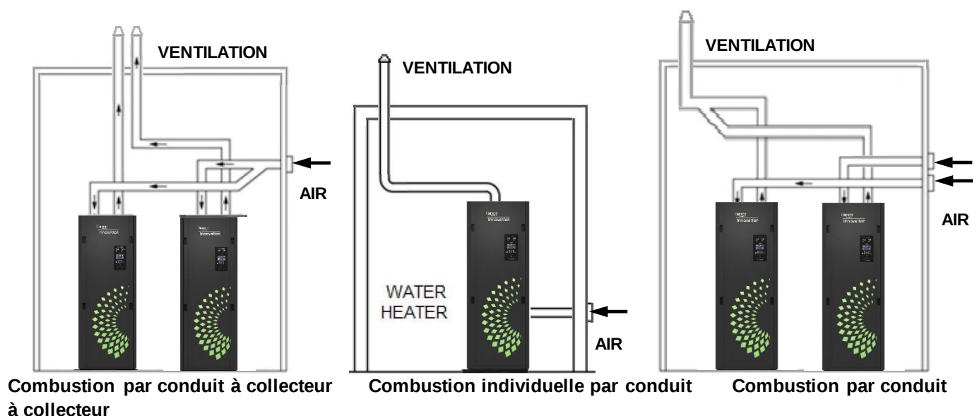
Figure 14d : Événements individuels – Installations ACCEPTABLES
