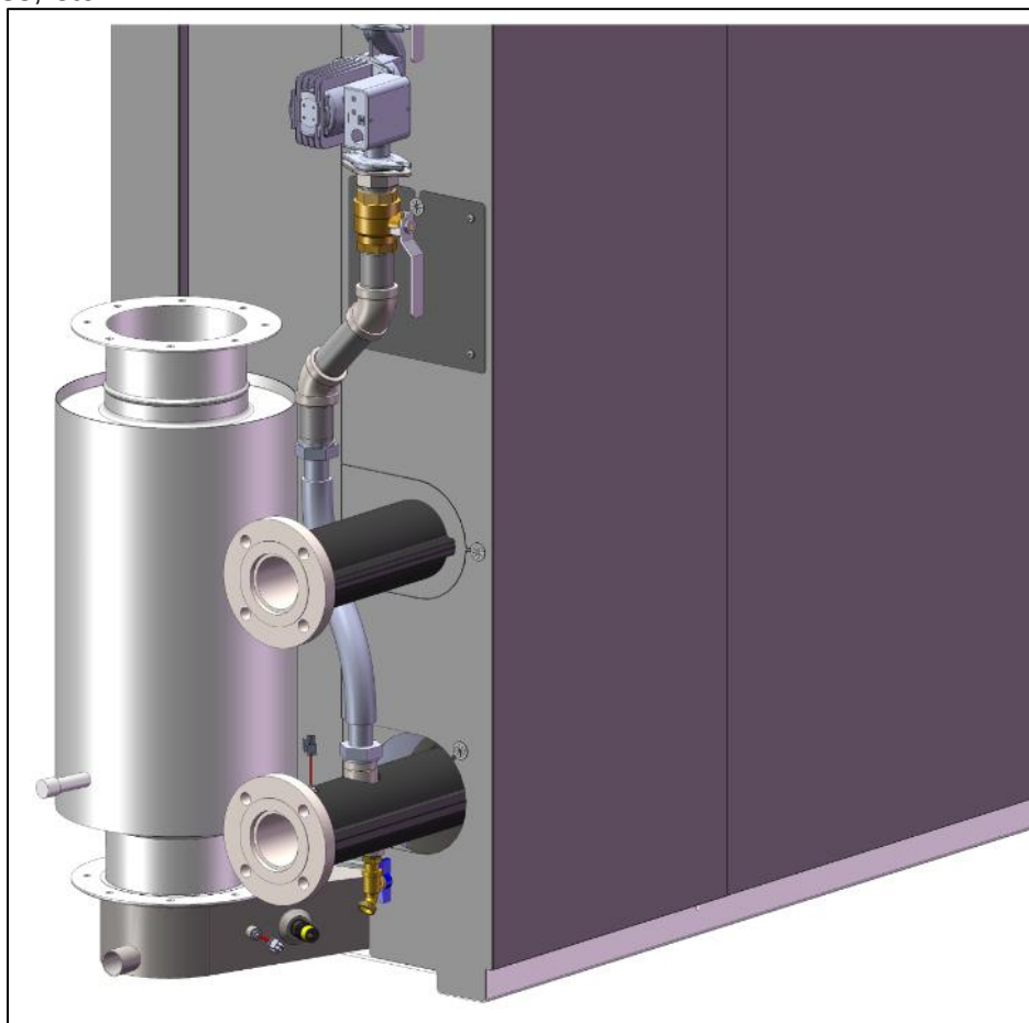
Figure 10-1: Échappement AERCO à bride Silencieux
