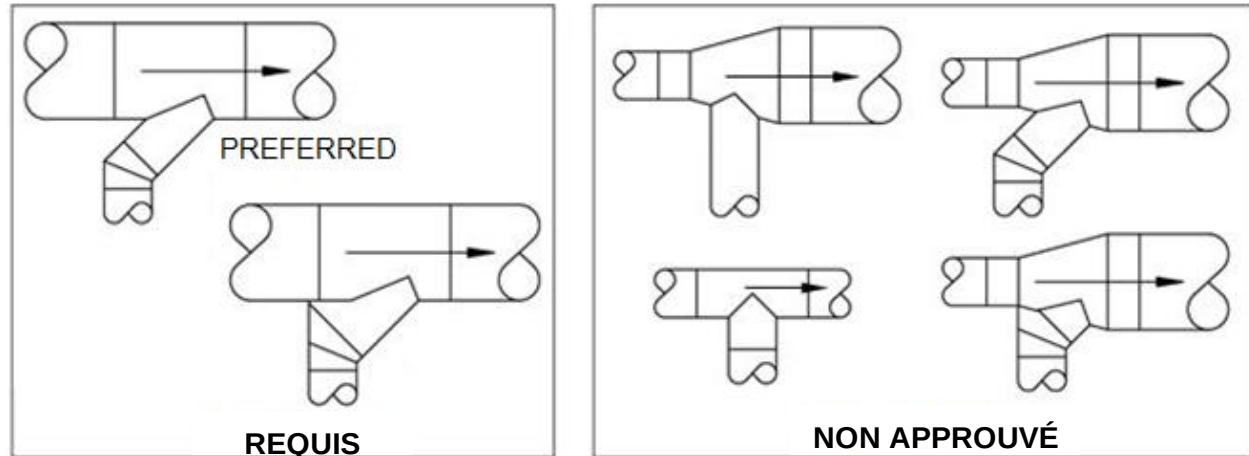
Figure 15c : Sections d'évent de transition requises
