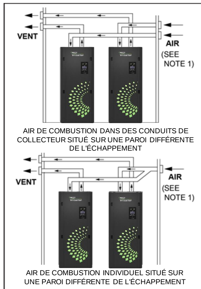
Figure 14b : Évents individuels – Installations acceptables
