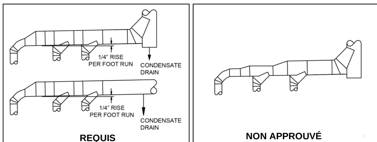
Figure 15d : Raccordement de l'unité à l'extrémité de la conduite d'évacuation
