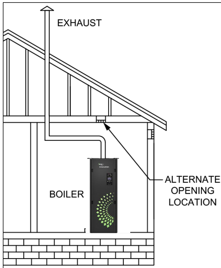
Figure 4-5: Tout l'air de combustion de l'extérieur jusqu'à Ouverture d'air de combustion simple
