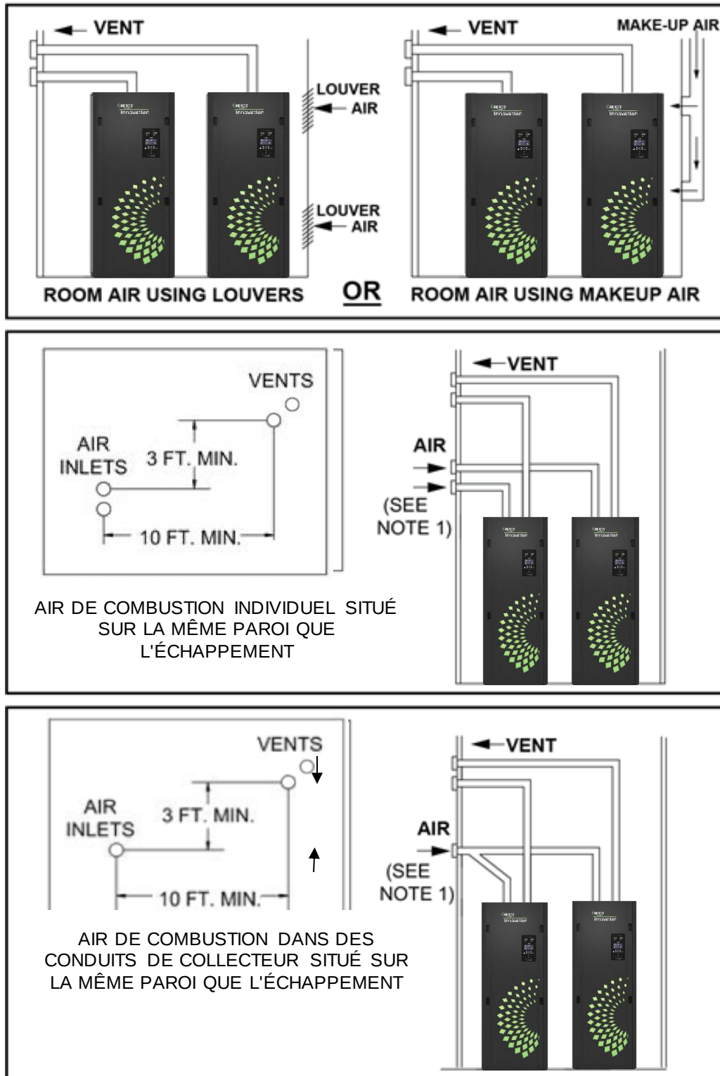
Figure 14a : Évents individuels – Installations privilégiées
