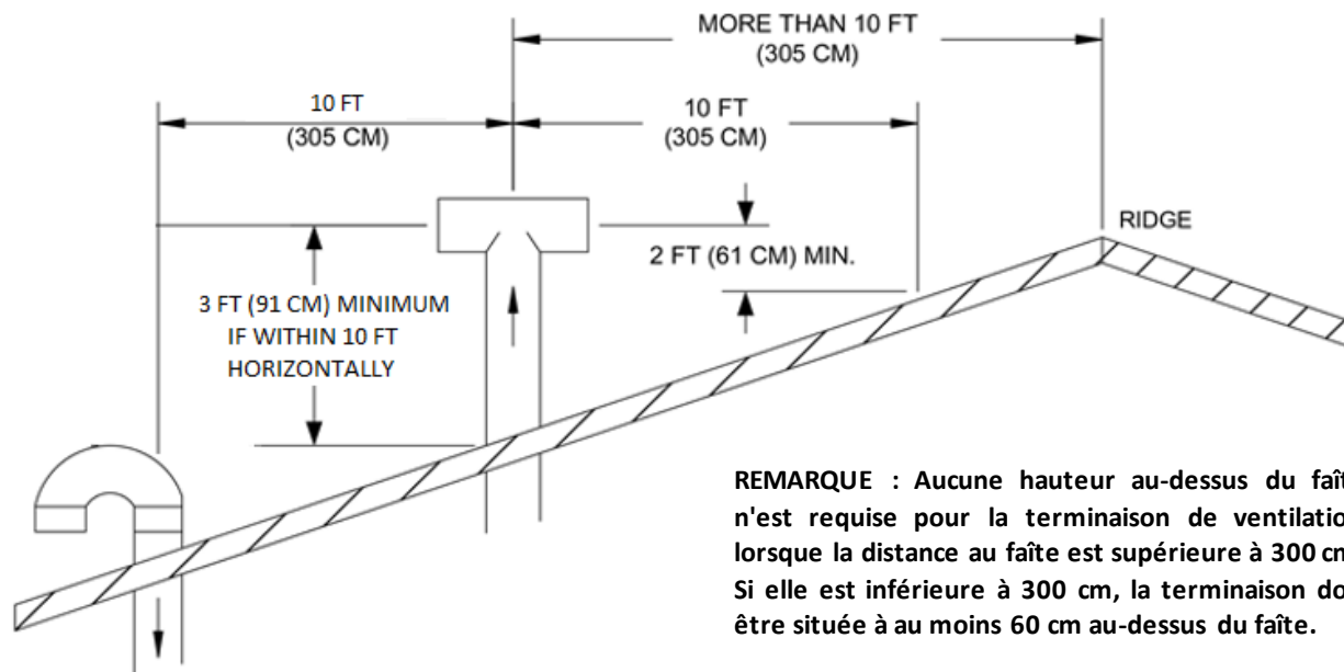
Figure 14f : Configuration acceptable de l'entrée et de la sortie d'air de combustion
