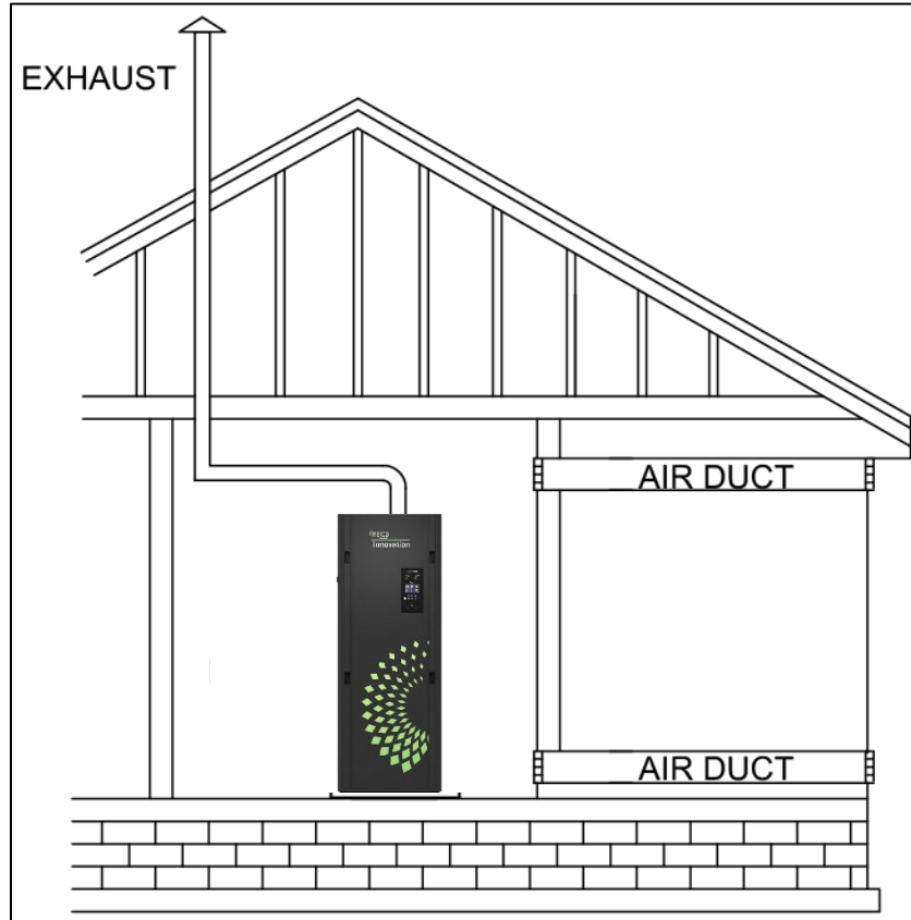
Figure 4-4: Tout l'air de combustion de l'extérieur par les conduits horizontaux
