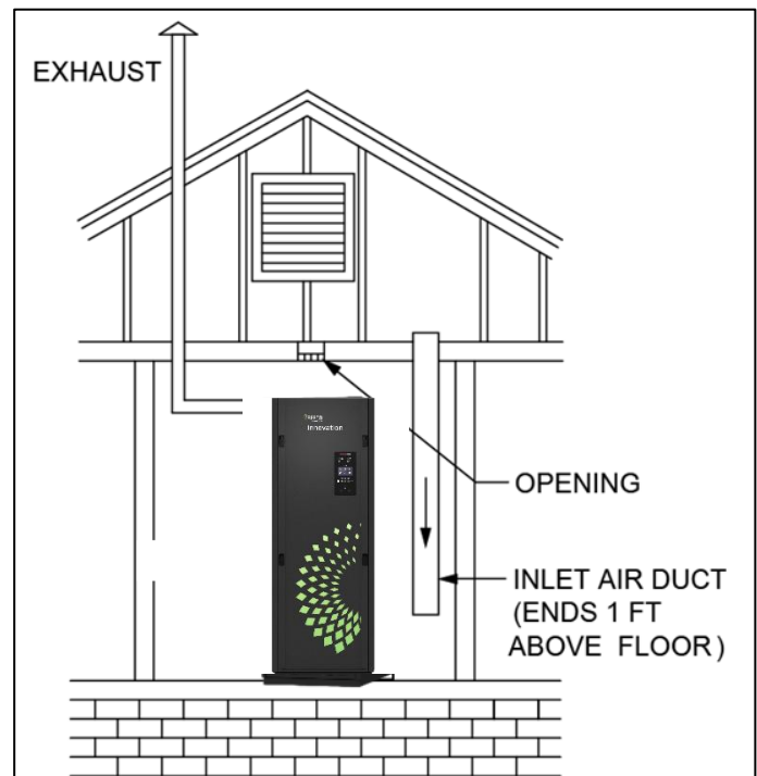
Figure 4-3: Tout l'air de combustion de l'extérieur - à travers le grenier ventilé
