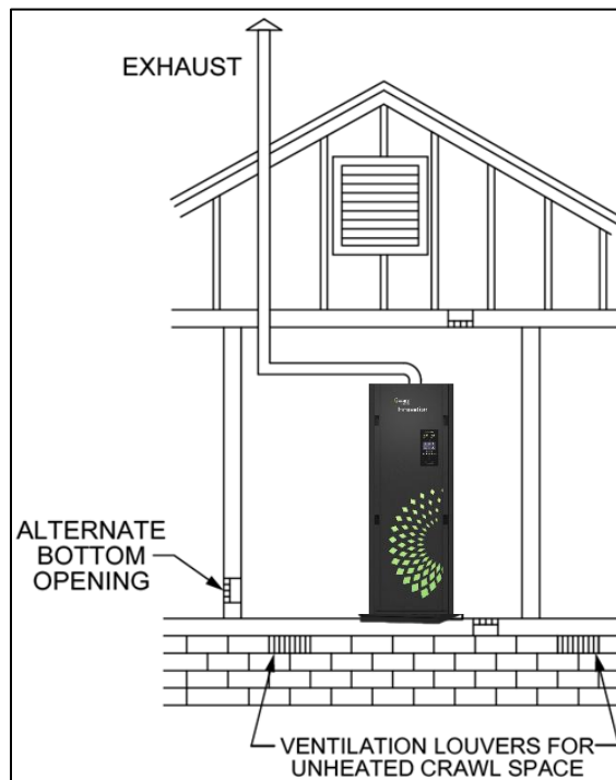
Figure 4-2: Tout l'air de combustion de l'extérieur - Air d'entrée du vide sanitaire ventilé et de l'air de sortie vers le grenier ventilé
