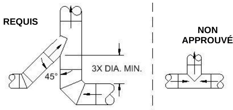
Figure 15b : Interconnexion requise des groupes d'unités
