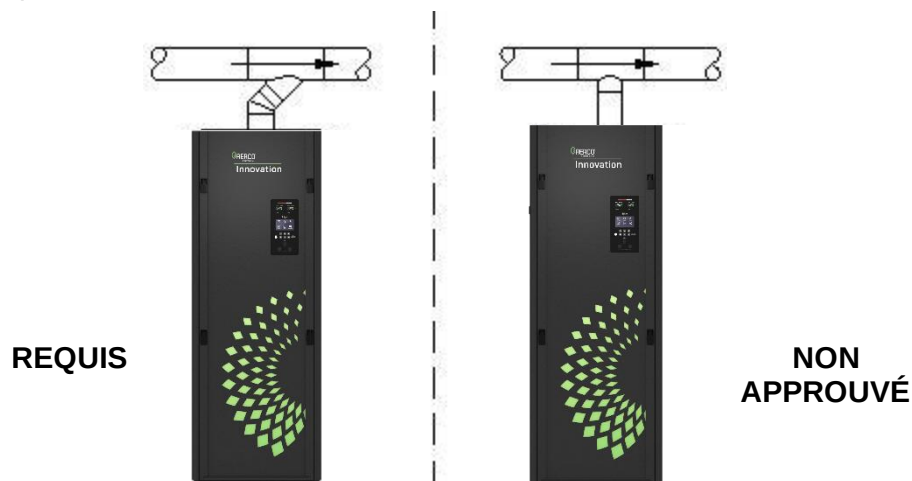
Figure 15a : Raccords requis à la culasse de l'évent commun
