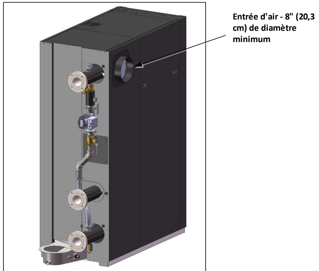
Figure 11 : Adaptateur d'entrée d'air arrière
