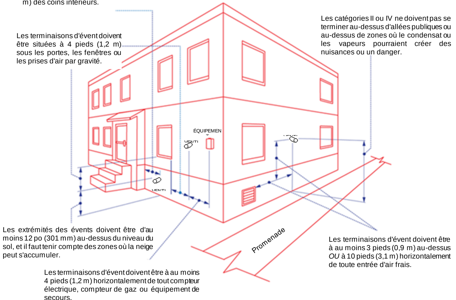
Figure 14e : Détermination de l'emplacement de la sortie d'évent
