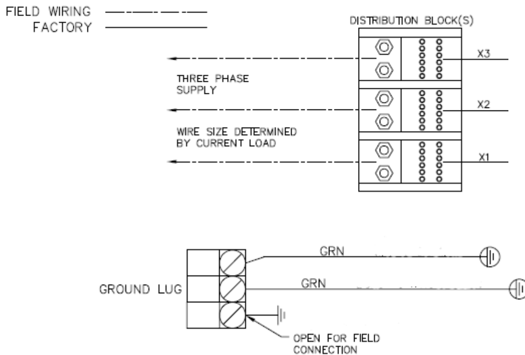
Figure 2a : Raccordements d'alimentation et de mise à la terre, BMK216 - 432
