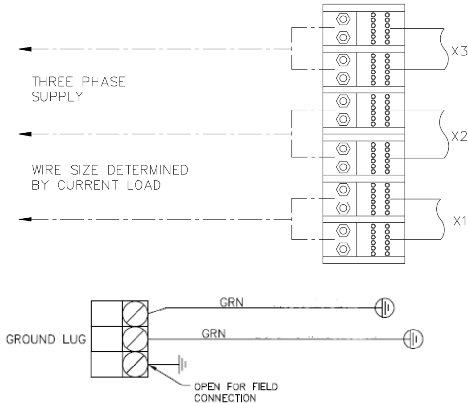
Figure 2b : Raccordements électriques et de mise à la terre, BMK 576 et 684
